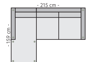
Texas 3-Divan Venstre/Høyre B:215 L:159 D:92 H:85 cm
