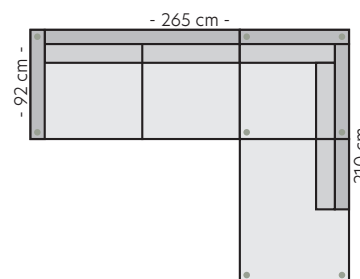
Texas 3HA Venstre/Høyre B:265 L:210 D:92 H:85 cm
